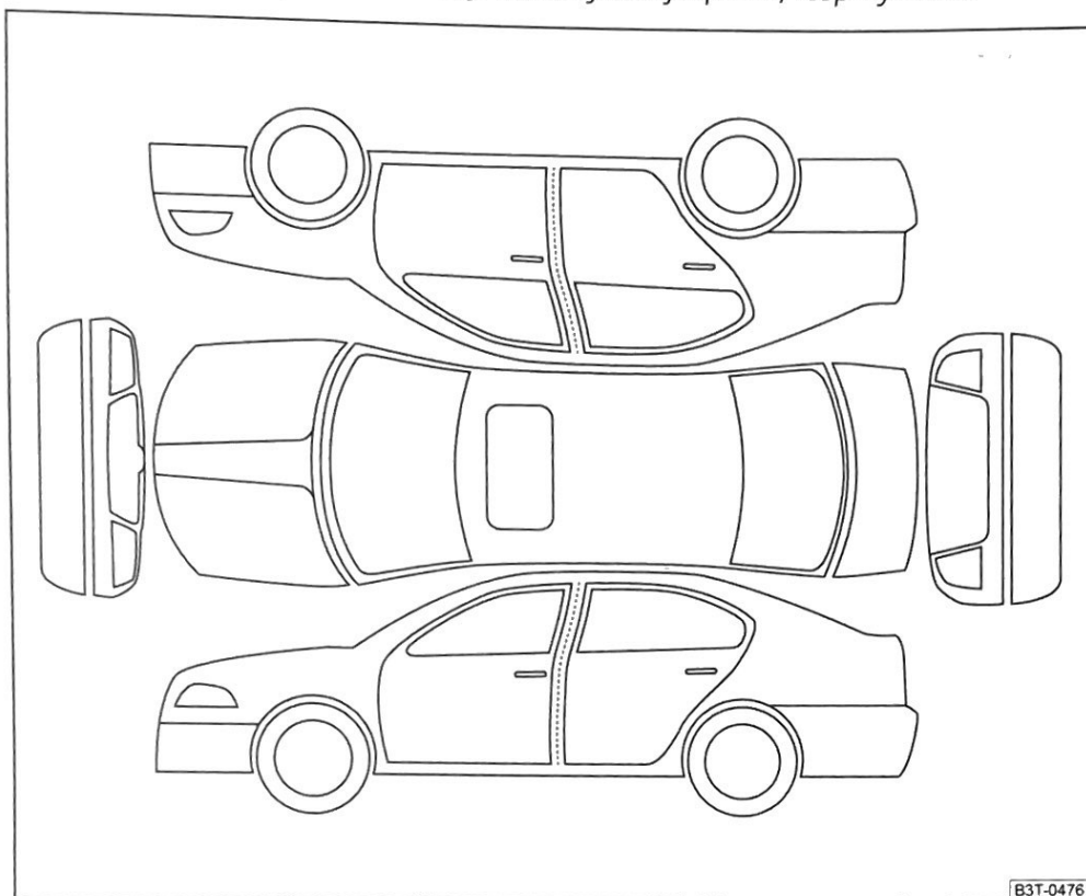
Obr. 3 Karoserie
